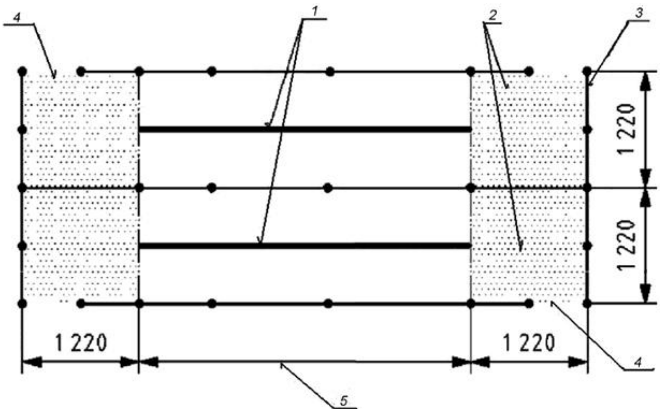
б) Параллельное размещение подвесных дорог
