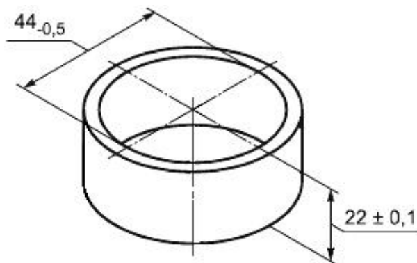
Рисунок Г.1 - Калибр
